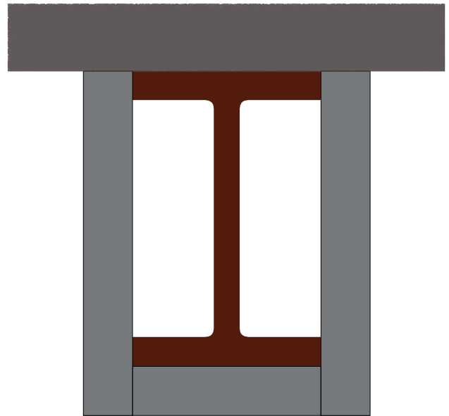
Indklædning af I-profil, bjælke 3 sidig. Det eksponerede areal beregnes som 2 \times \text{profilets højde} + 1 \times \text{profilets bredde} .
