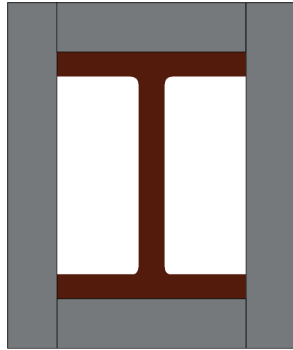
Indklædning af HEB bjælke 4 sidig. Det eksponerede areal beregnes som 2 \times \text{profilens højde} + 2 \times \text{profilens bredde} .
